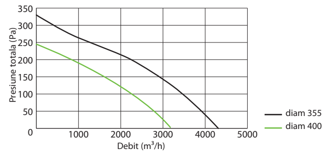
Canal Fast isolé 355 et 400
