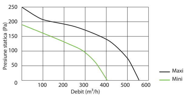
Canal Fast isolé 150
