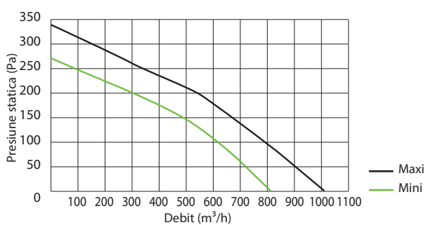
Canal Fast isolé 250
